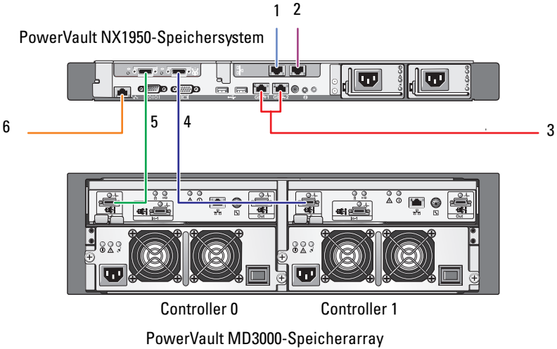
Abbildung 2-1. Einzelknotenkonfiguration
